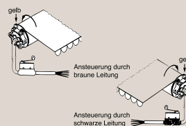
HiPro-Kabel mit externem Grenztaster
